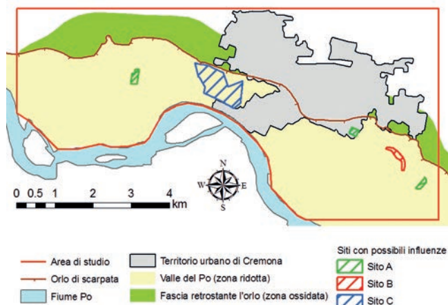
Fig. 2 - Area di studio con la zona ridotta (valle del Po) e ossidata (fascia retrostante l'orlo di scarpata) e i tre siti con possibili influenze antropiche sulle concentrazioni di As, Fe e Mn.
