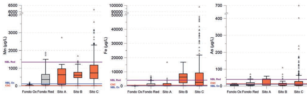
Fig. 3 - Box-plot delle serie storiche di Mn, Fe ed As misurate nell'acquifero F suddivise in fondo naturale (zona ossidata e ridotta), in grigio, e in siti con possibili influenze antropiche (sito A, B e C), in rosso, e con i rispettivi NBL e CSC.
