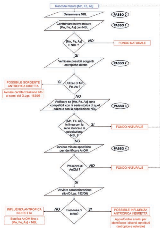
Fig. 4 - Diagramma di flusso della procedura proposta per la gestione di potenzialmente contaminazioni da As, Fe e Mn nella bassa Pianura Padana.
