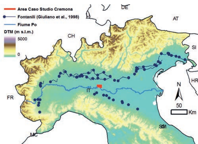
Fig. 1 - Inquadramento geografico dell'area del caso studio di Cremona con ubicazione della fascia dei fontanili (Giuliano et al., 1998).
